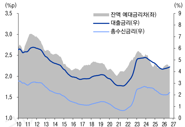
그림5 잔액기준 예대금리차
