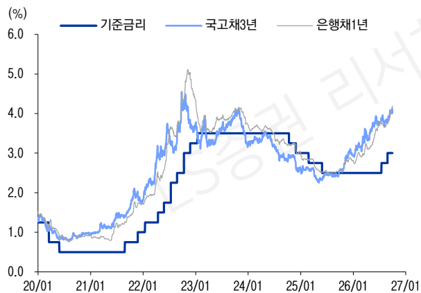
그림2 시장금리 추이
